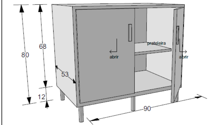
Balcão dimensão 90x80x53cm.
