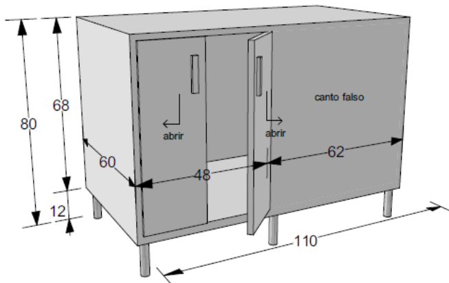
Balcão de Canto em MDF 110x80x60cm s.
