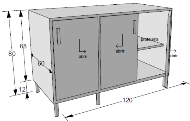
Balcão em MDF, dimensão 120x80x60cm
