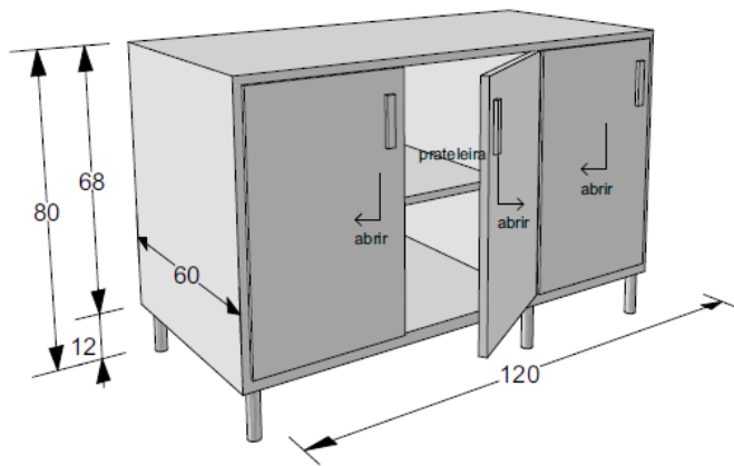
Balcão dimensão 120x80x60cm.
