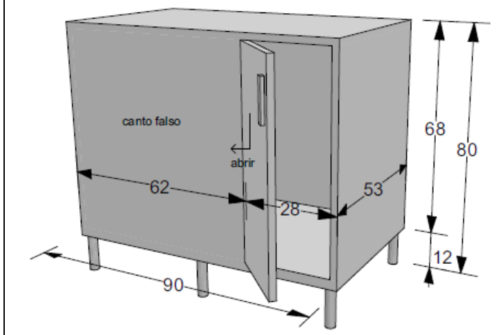
Balcão de Canto dimensão 90x80x53cm.
