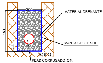
DRENO PROFUNDO DISPOSITIVO DE DRENAGEM DPS 08
