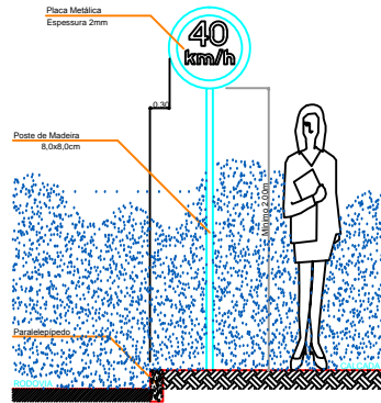
DETALHE 01 POSICIONAMENTO DE PLACAS EM RELAÇÃO AO MEIO-FIO E NÍVEL DO PASSEIO
