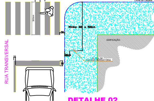
DETALHE 02 POSICIONAMENTO DA PLACA DE PARADA OBRIGATORIA EM RELAÇÃO A ESQUINA E FAIXA PARA PEDESTRES
