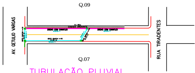
TUBULAÇÃO PLUVIAL Escala: _____ 1:1.000
