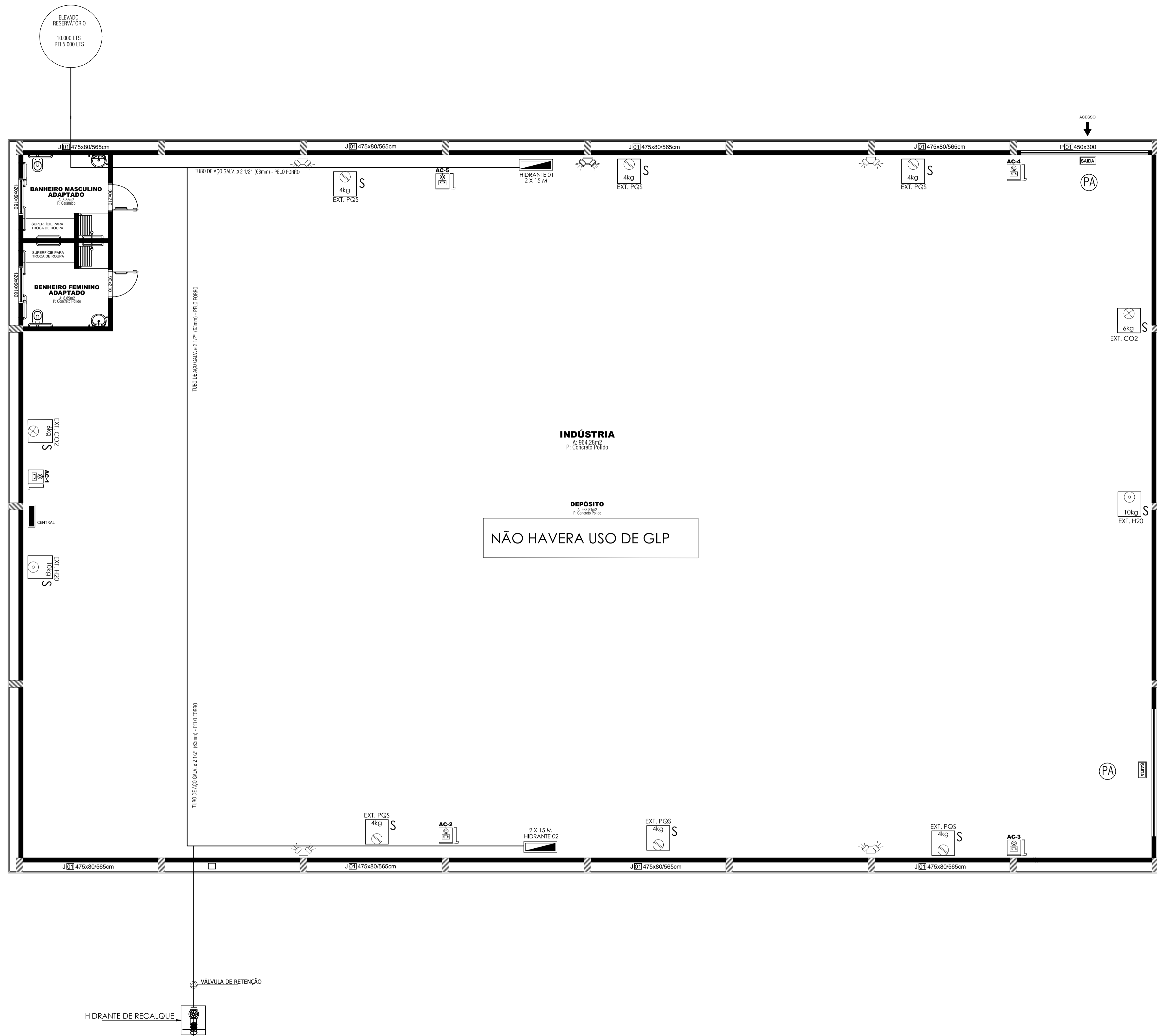
PLANTA BAIXA - SISTEMA PREVENTIVO ESCALA 1/75
