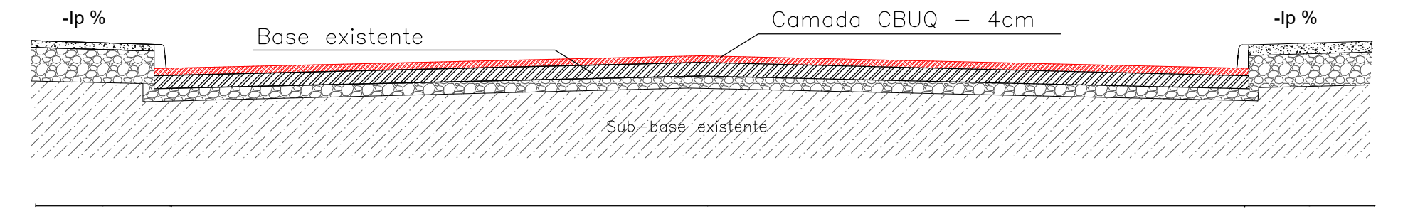
DETALHES DA PAVIMENTAÇÃO TRECHO 2
