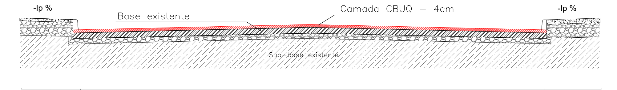
DETALHES DA PAVIMENTAÇÃO TRECHO 1
